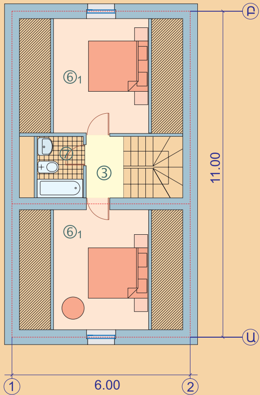
ԶԵՂՆԱՀԱՐԿԻ ՀԱՏԱԿԱԳԻԾ
