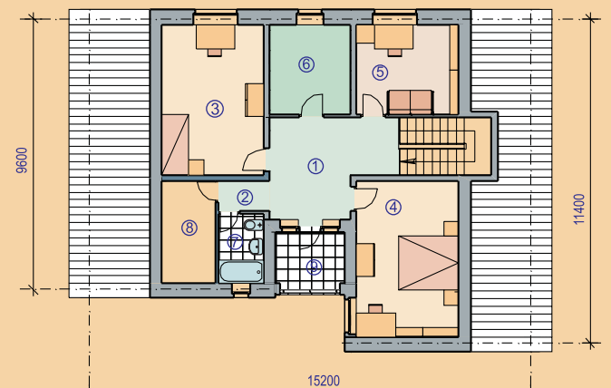
ԵՐԿՐՈՐԴ ՀԱՐԿԻ ՀԱՏԱԿԱԳԻԾ
