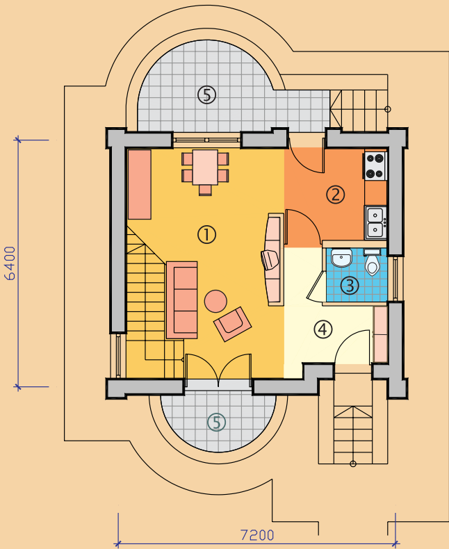
ԱՌԱՋԻՆ ՀԱՐԿԻ ՀԱՏԱԿԱԳԻԾ
