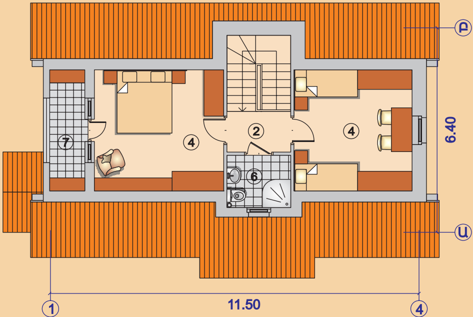
Մանսարդային հարկի հատակագիծ
