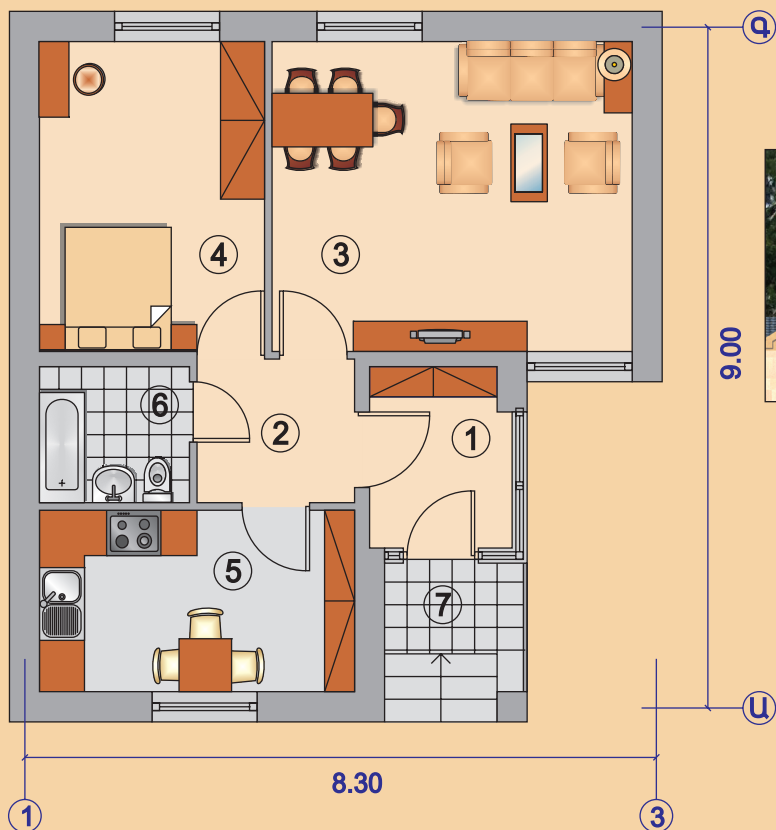
ՀԱՐԿԻ ՀԱՏԱԿԱԳԻԾ
