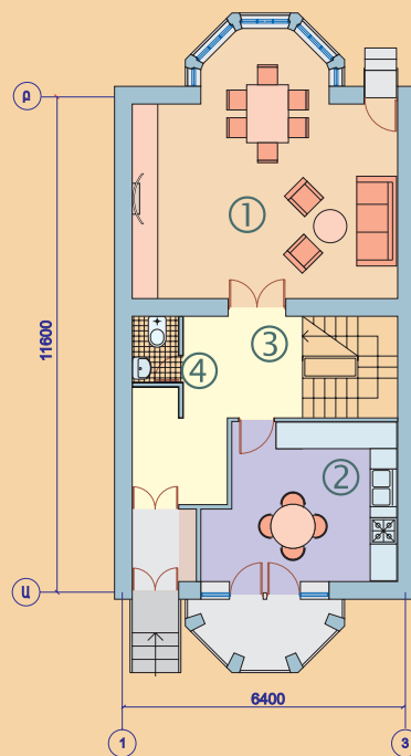
ԱՌԱՋԻՆ ՀԱՐԿԻ ՀԱՏԱԿԱԳԻԾ
