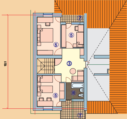
ԵՐԿՐՈՐԴ ՀԱՐԿԻ ՀԱՏԱԿԱԳԻԾ
