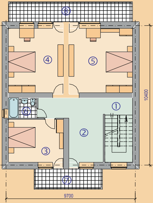
ԵՐԿՐՈՐԴ ՀԱՐԿԻ ՀԱՏԱԿԱԳԻԾ
