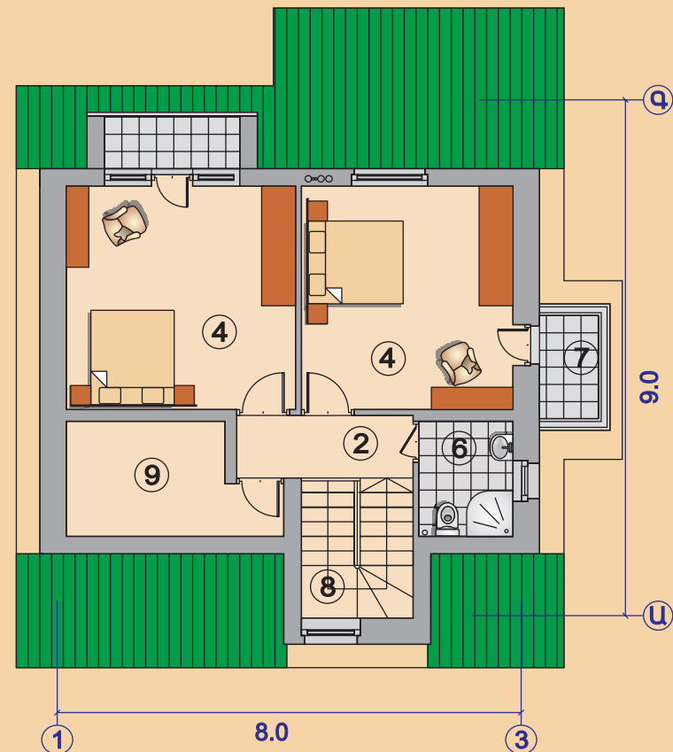
Ձեղնահարկի հատակագիծ
