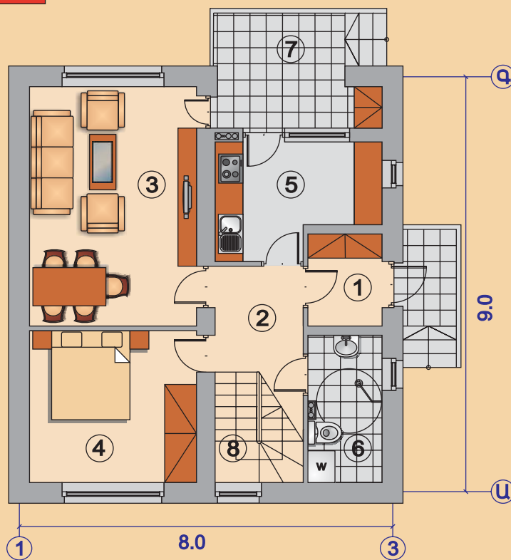
Առաջին հարկի հատակագիծ
