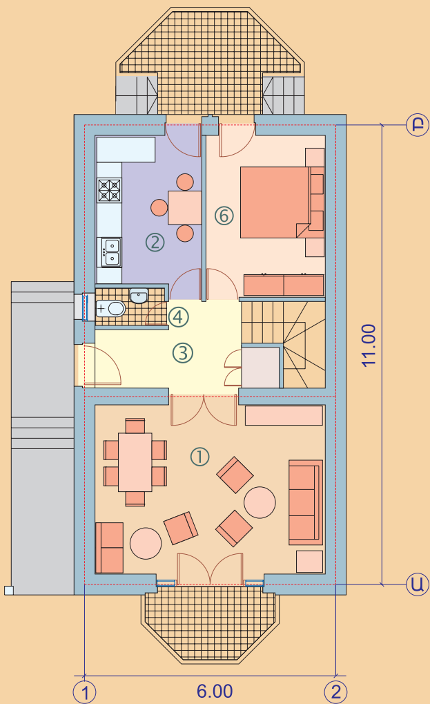
ԱՌԱՋԻՆ ՀԱՐԿԻ ՀԱՏԱԿԱԳԻԾ
