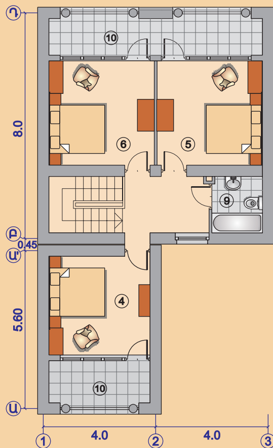
ԵՐԿՐՈՐԴ ՀԱՐԿԻ ՀԱՏԱԿԱԳԻԾ
