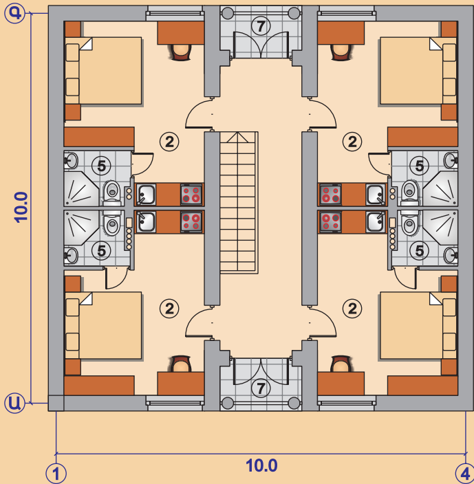
ԵՐԿՐՈՐԴ ՀԱՐԿԻ ՀԱՏԱԿԱԳԻԾ
