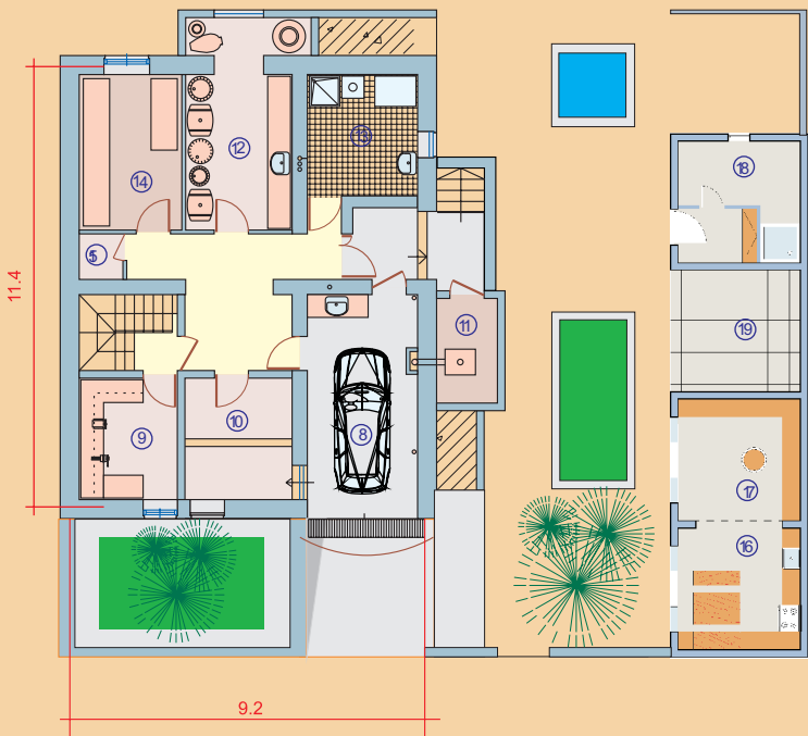
ԿԻՍԱՆԿՈՒՂԱՅԻՆ ԵՎ ԲԱՎԱՅԻՆ ՏՆՏԵՍԱԿԱՆ ՇԻՆՈՒԹՅՈՒՆՆԵՐԻ ՀԱՏԱԿԱԳԻԾ
