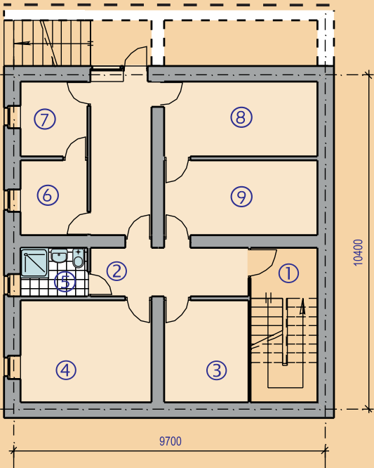
ՆԿՈՒՂԱՅԻՆ ՀԱՐԿԻ ՀԱՏԱԿԱԳԻԾ
