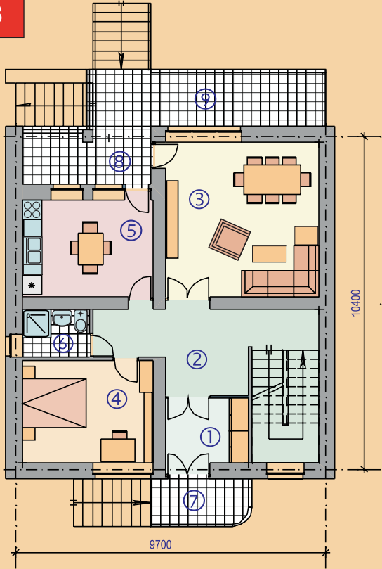
ԱՌԱՋԻՆ ՀԱՐԿԻ ՀԱՏԱԿԱԳԻԾ
