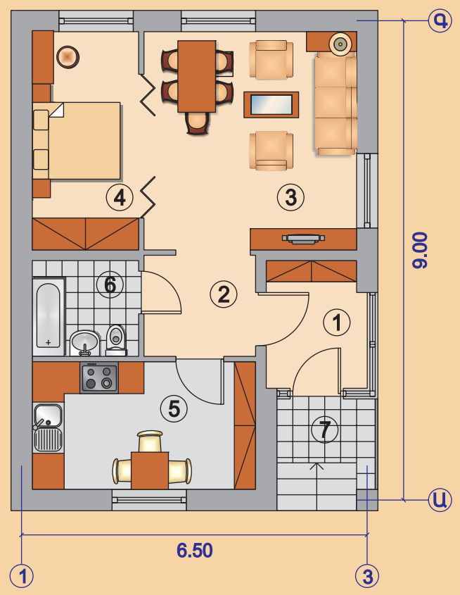
ԱՌԱՋԻՆ ՀԱՐԿԻ ՀԱՏԱԿԱԳԻԾ
