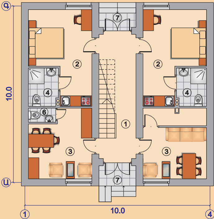
ԱՌԱՋԻՆ ՀԱՐԿԻ ՀԱՏԱԿԱԳԻԾ
