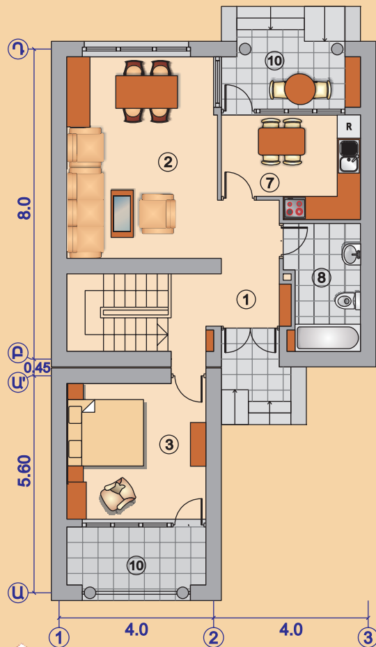
ԱՌԱՋԻՆ ՀԱՐԿԻ ՀԱՏԱԿԱԳԻԾ
