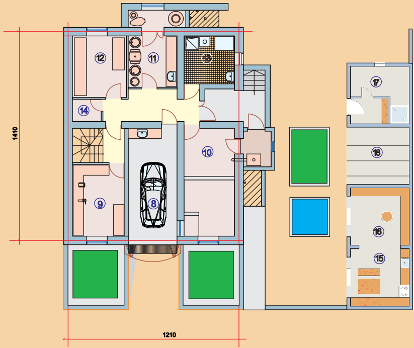
ԿԻՍԱՆԿՈՒՂԱՅԻՆ ԵՎ ԲԱԿԱՅԻՆ ՏՆՏԵՍԱԿԱՆ ՇԻՆՈՒԹՅՈՒՆՆԵՐԻ ՀԱՏԱԿԱԳԻԾ
