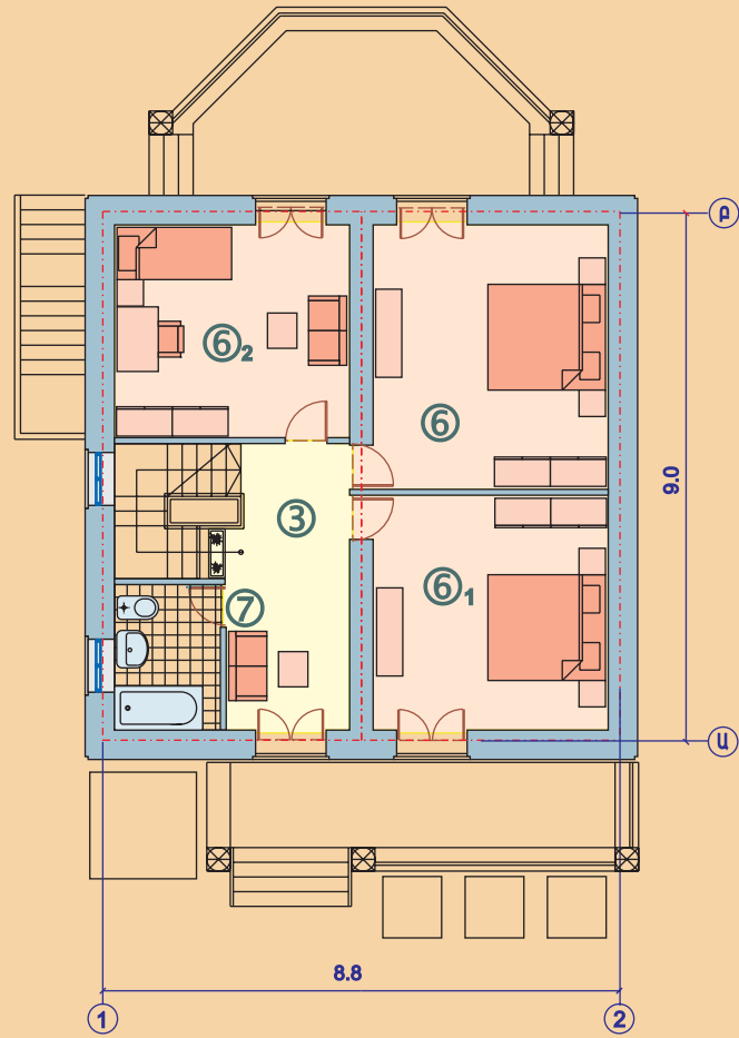
ՁԵՂՆԱՀԱՐԿԻ ՀԱՏԱԿԱԳԻԾ
