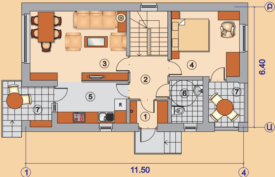
Առաջին հարկի հատակագիծ
