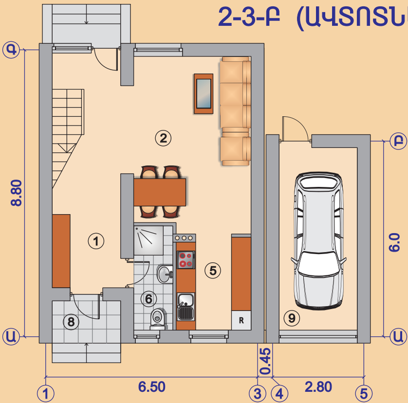
Առաջին հարկի հատակագիծ
