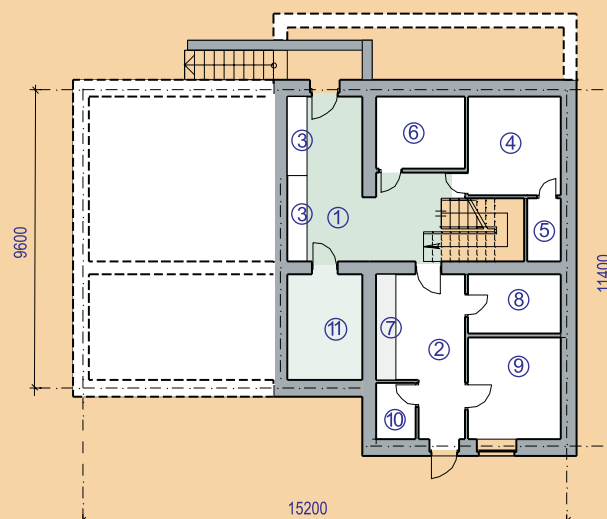
ՆԿՈՒՂԱՅԻՆ ՀԱՐԿԻ ՀԱՏԱԿԱԳԻԾ
